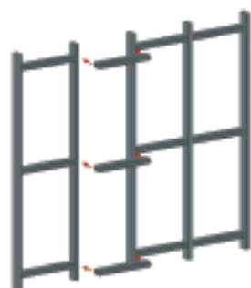
Beispiel einer Vorhangfassade in Pfosten-Riegel-Bauweise.
