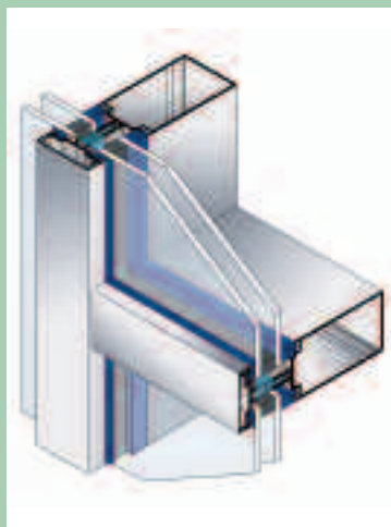
Prinzipdarstellung des Alcoa-Systems AA100 Riegel/Riegel.
